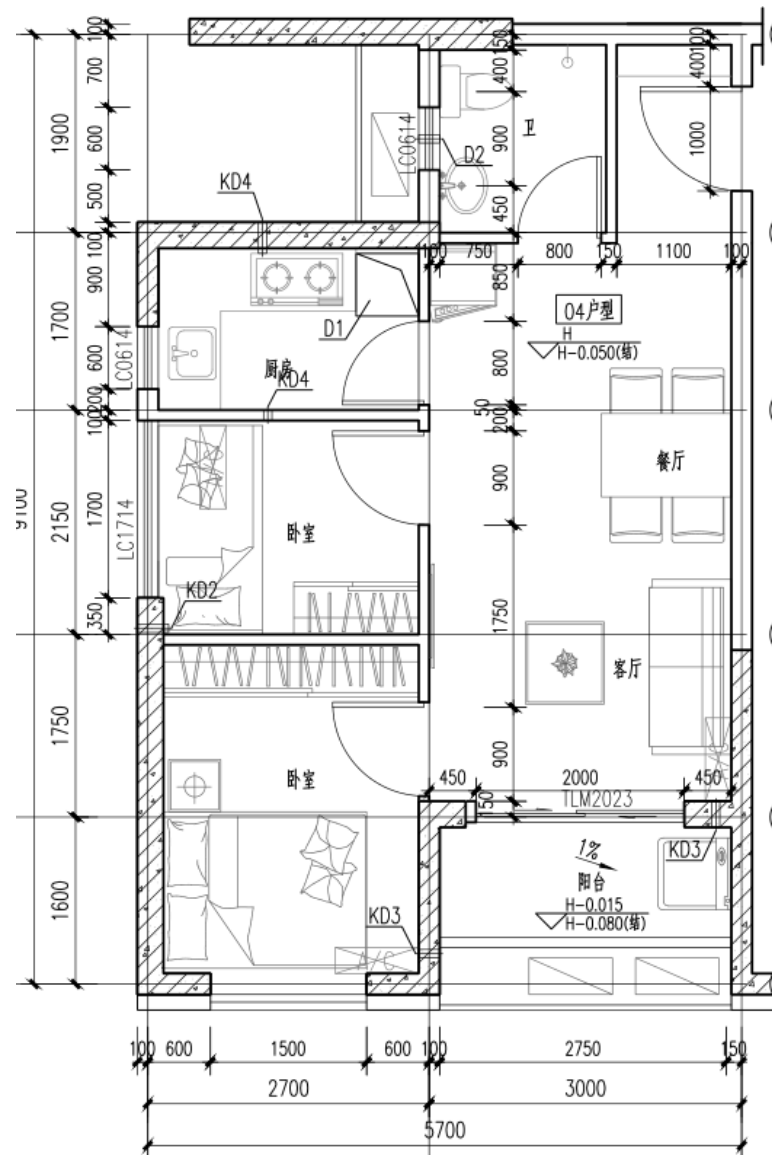
D-2户型
