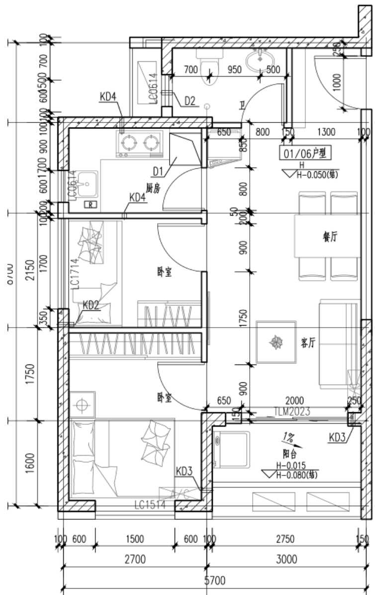
D-1户型
